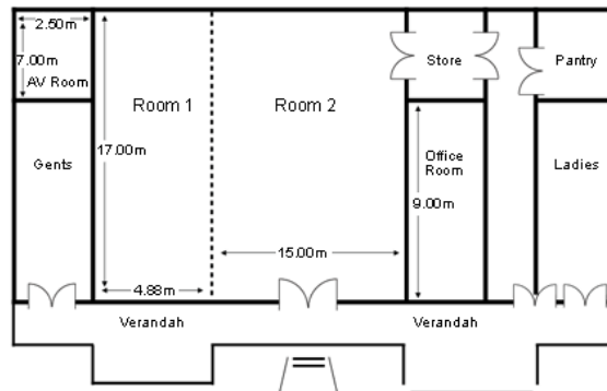
컨퍼런스 홀 배치도
